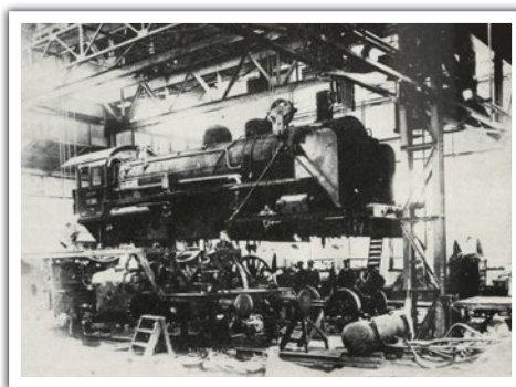
1900: Einachsen einer Dampflokomotive - S102 Lok am Kran, BR17
